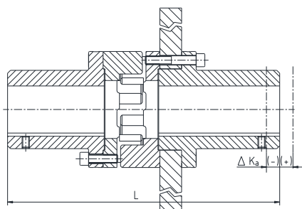
Axiella förskjutningar
