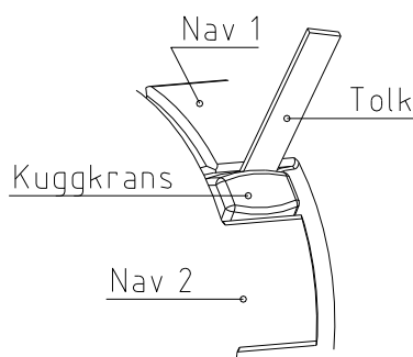
Bild 10: Kontroll av slitagegränsen
