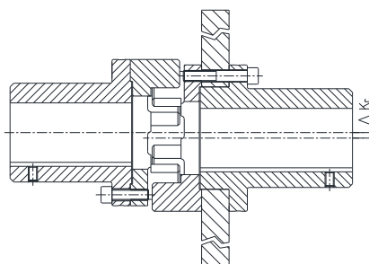
Radiella förskjutningar
