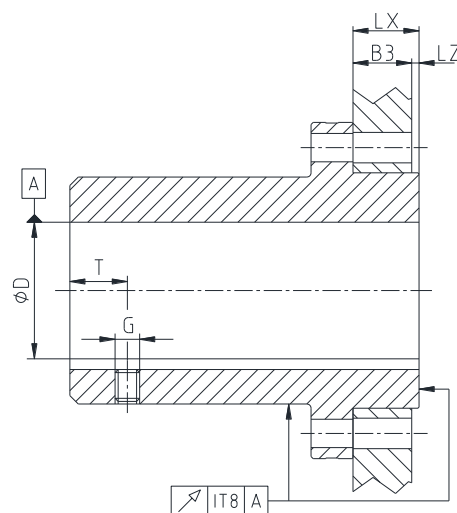
Bild 3: Rund- och plangångsnoggrannhet
