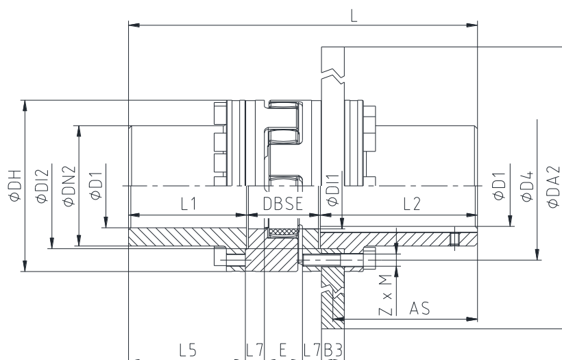
Bild 1: ROTEX®, Utförande AFN-SB spec.
