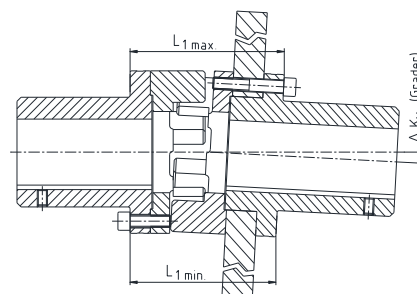
Vinkelförskjutningar
