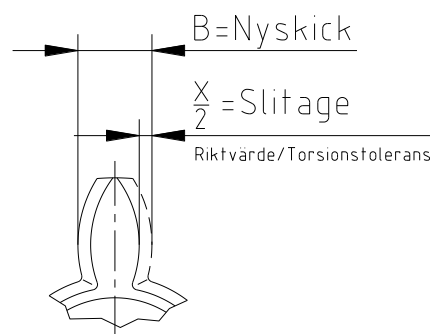
Bild 11: Kuggkransslitage
